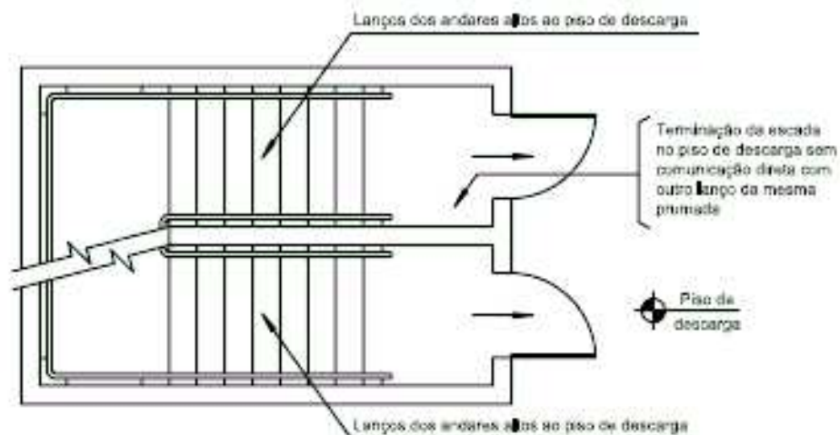
Figura 3 – Segmentação das escadas no piso de descarga
