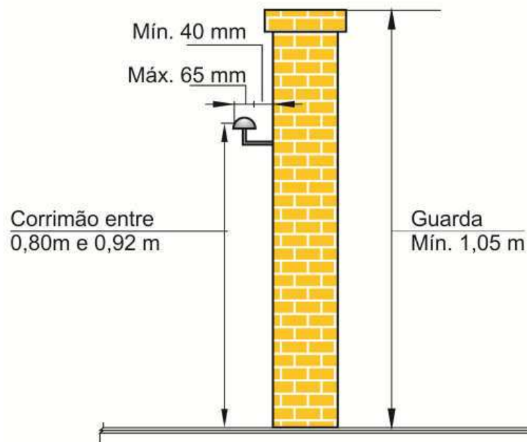
Figura 14 – Dimensões de guardas e corrimãos
