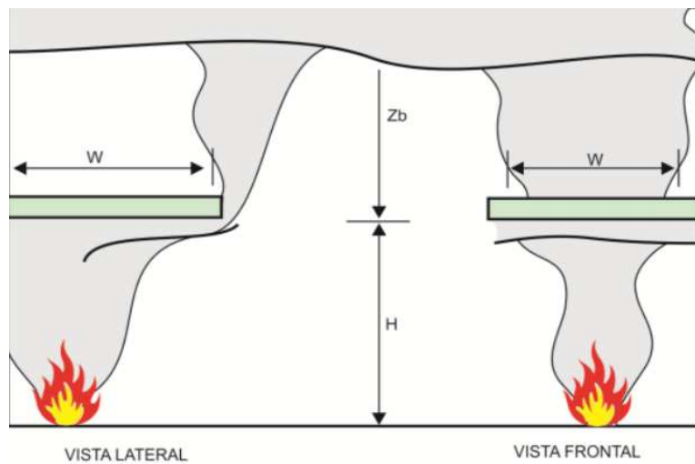
Figura 18 - Máxima corrente volumétrica por ponto de sucção ou ventilador individual
